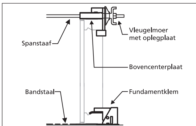
Schematische opbouw
