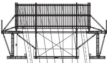
Utilisation comme coffrage grim pant
