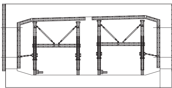
Utilisation comme chariot de coffrage composite
