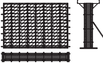
Utilisation comme coffrage de mur
