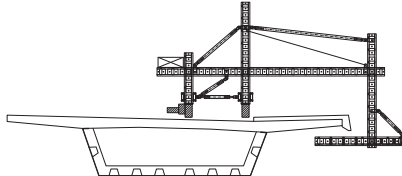
Utilisation comme coffrage de cuvette
