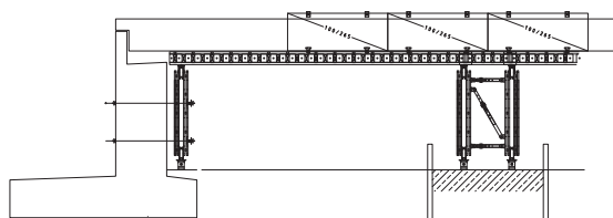
Utilisation comme échafaudage d'encorbellement
