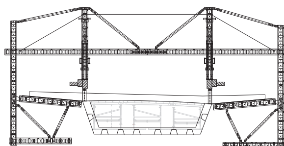
Utilisation comme chariot de coffrage composite
