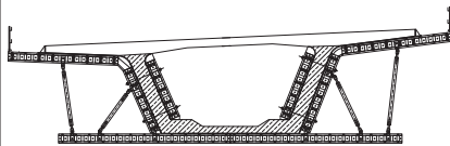
Inzet als trogbekisting
