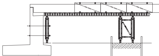
Inzet als ondersteuningsconstructie
