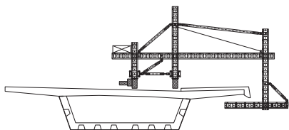
Inzet als werkbordes
