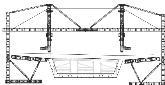
Bekisting voor brugconstructie
